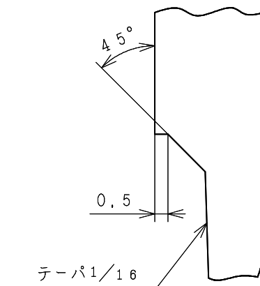
A部詳細
